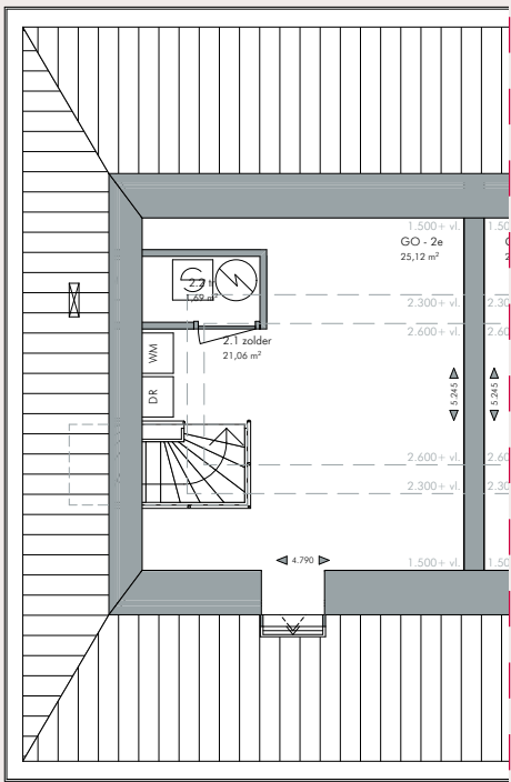
tweede verdieping
