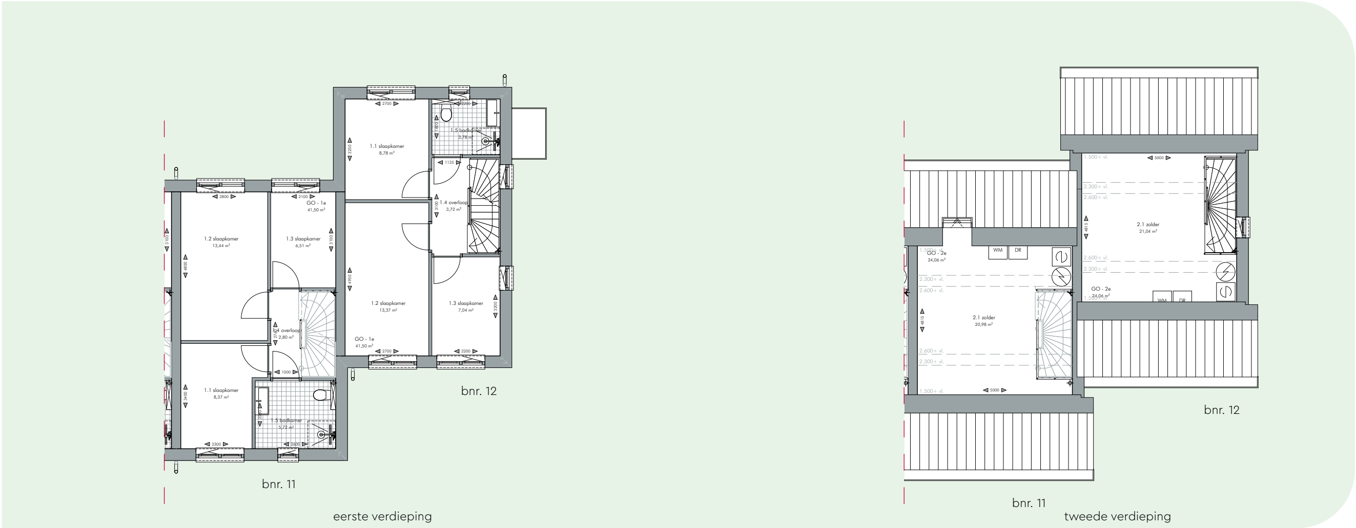
plattegrond bnr. 7 t/m 10 gelijk aan bnr. 11 bnr. 7 eindwoning,w met buitenmuur
