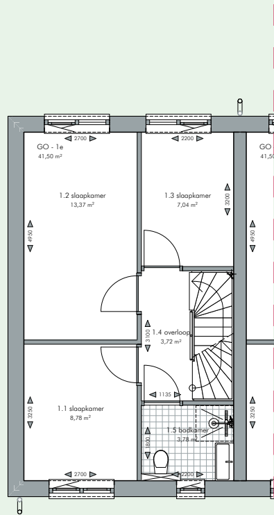
eerste verdieping
