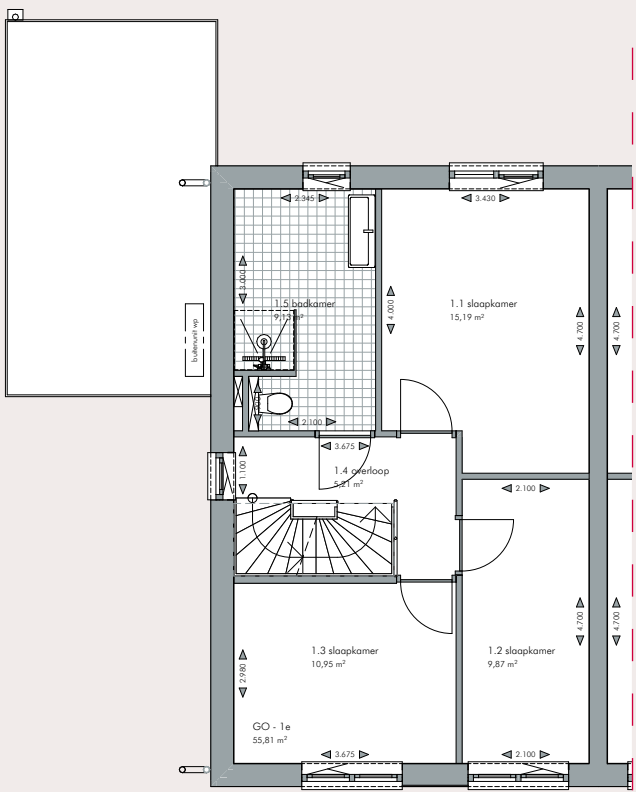
eerste verdieping
