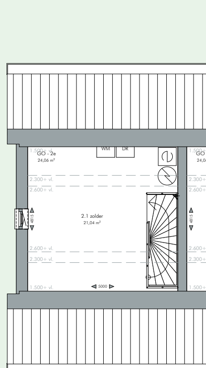
tweede verdieping
