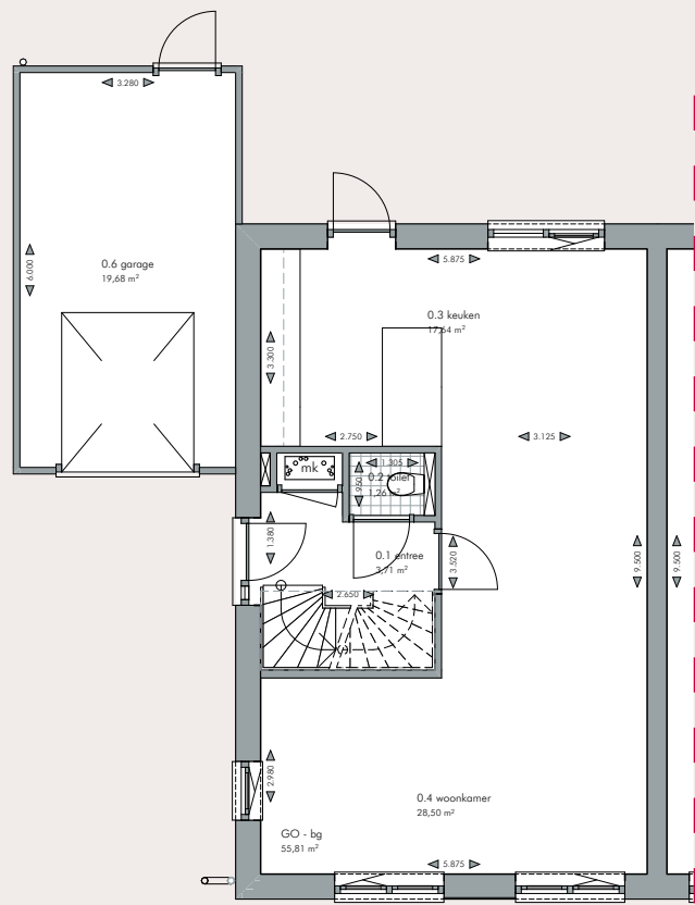
begane grond
