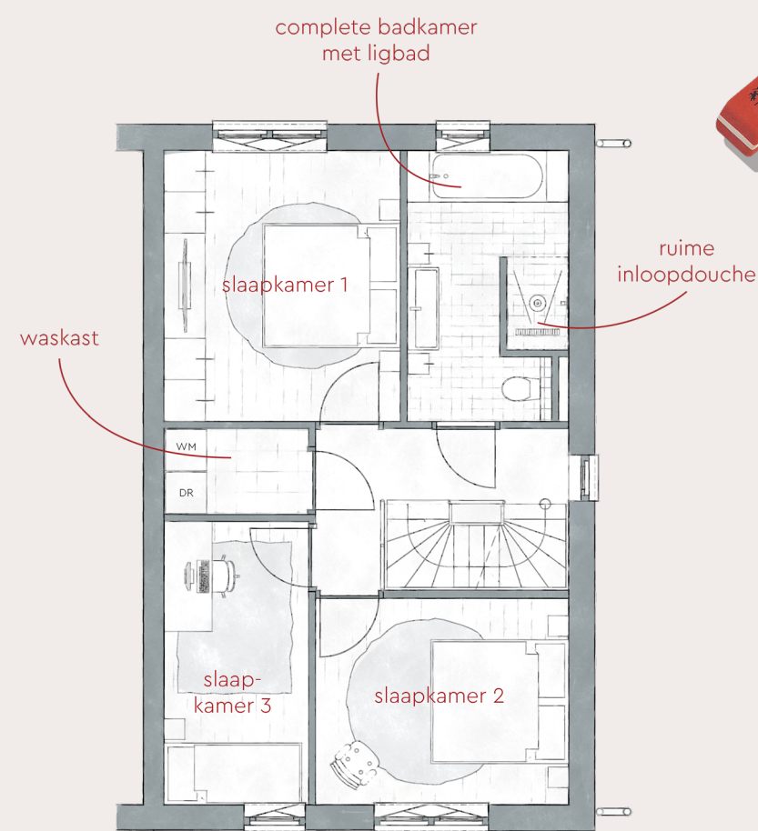
eerste verdieping
