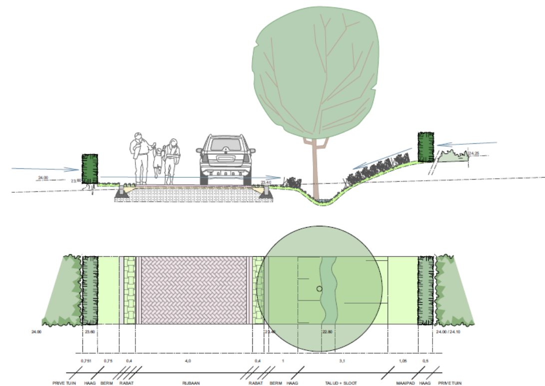
doorsnede rijbaan
