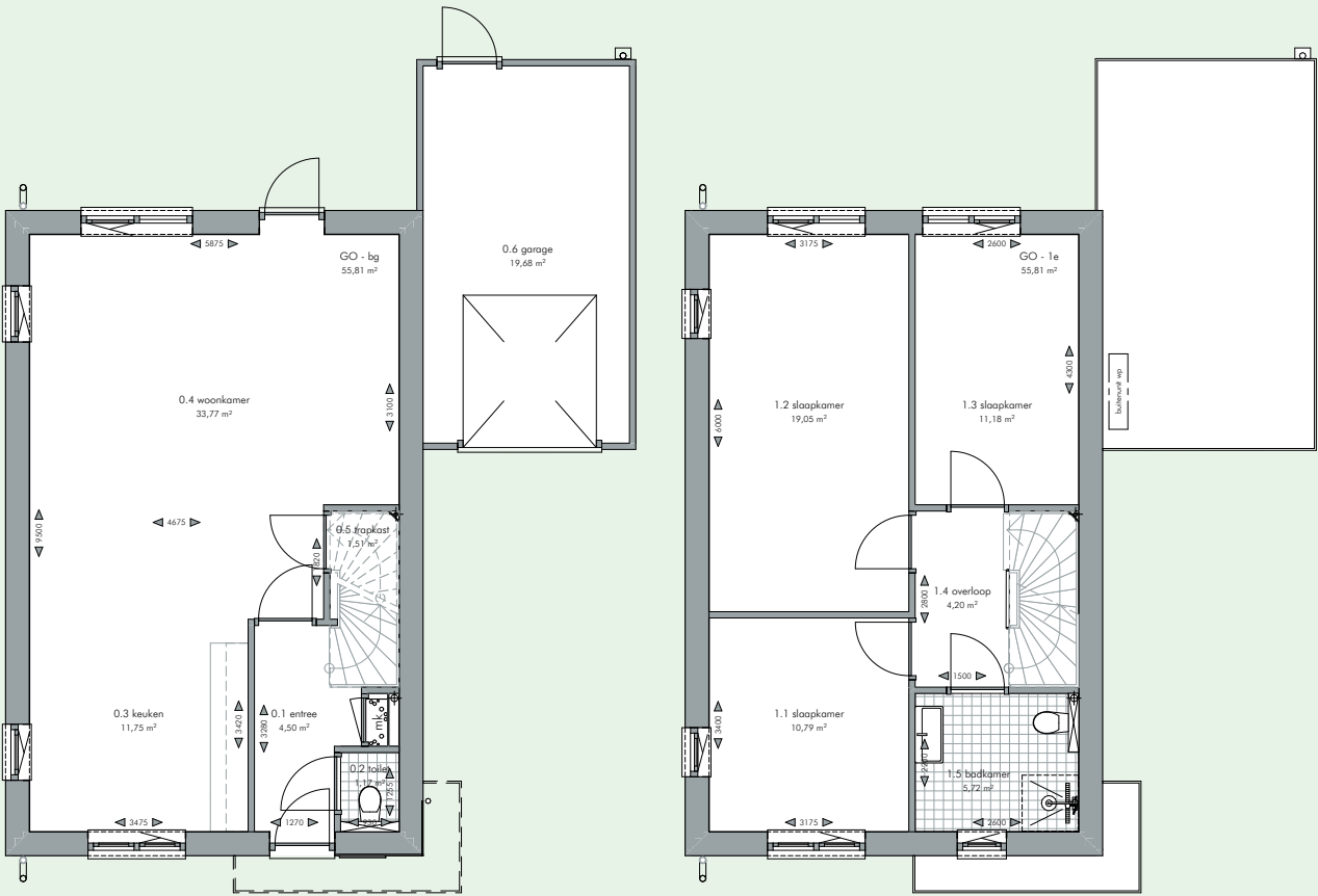
begane grond
